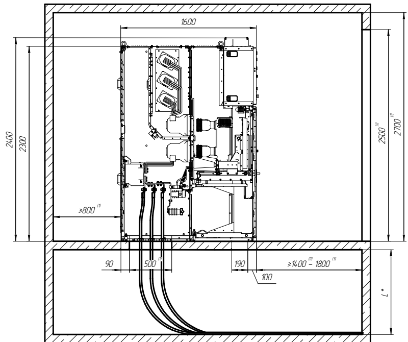
Установка над кабельным полуэтажом ячейки КРУ-СВЭЛ-К-1.4 глубиной 1600 мм
