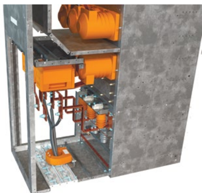
КРУ-СВЭЛ двустороннего обслуживания
